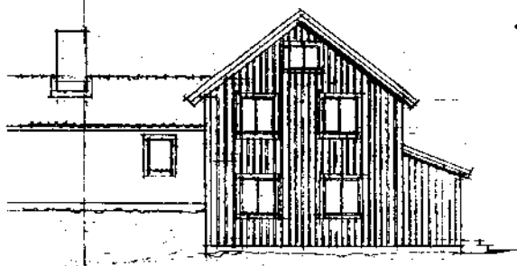
FASAD NÖT NORR
